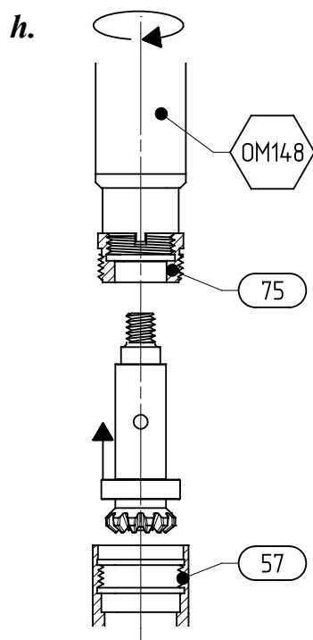
(démont. M180 arbre inter)
