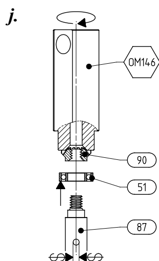
(démont. M180 pignon outil)
