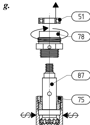
(démont. M180 manchon)
