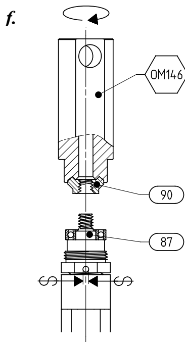
(démont. M180 pignon moteur)
