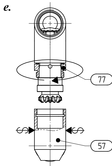
(démont. M180 corps moteur)
